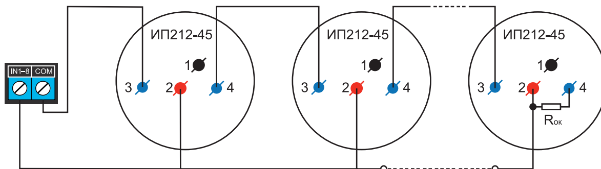
Рисунок 3. Схема подключения ИП212-45 к пожарному входу NV 2108 только с окончательным резистором
