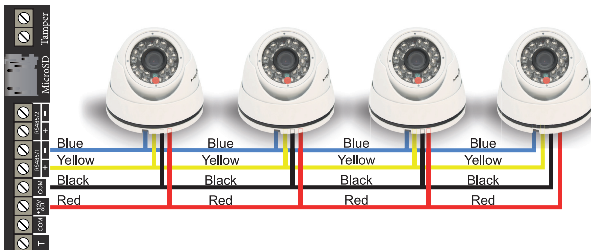
Рисунок 7. Подключение камер NV DOM 485-28IR к NV 2108
