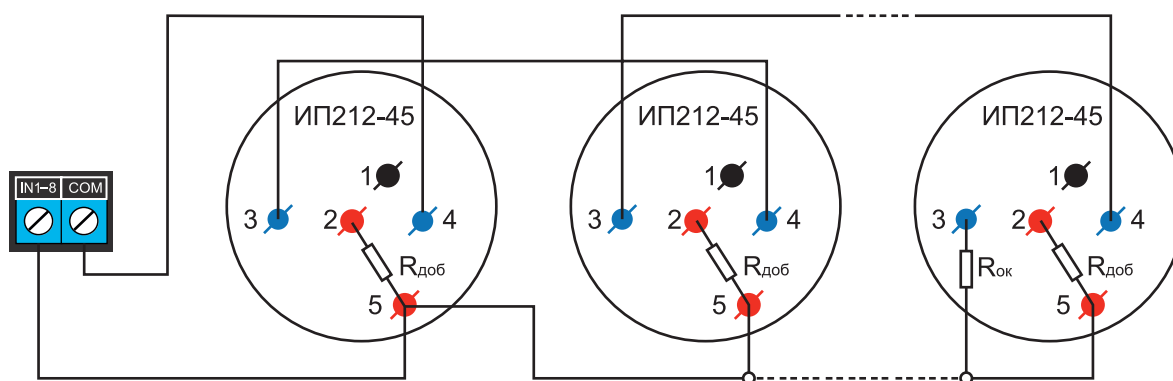
Рисунок 2. Схема подключения ИП212-45 к пожарному входу NV 2108 с добавочными и с окончечным резисторами
