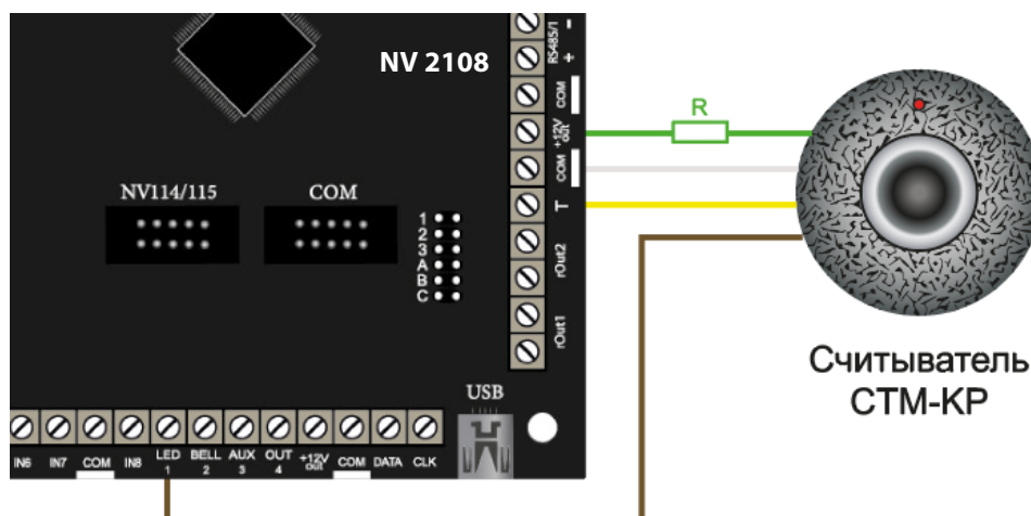
Рисунок 5. Схема подключения на примере ТМ считывателя CTM-KT
